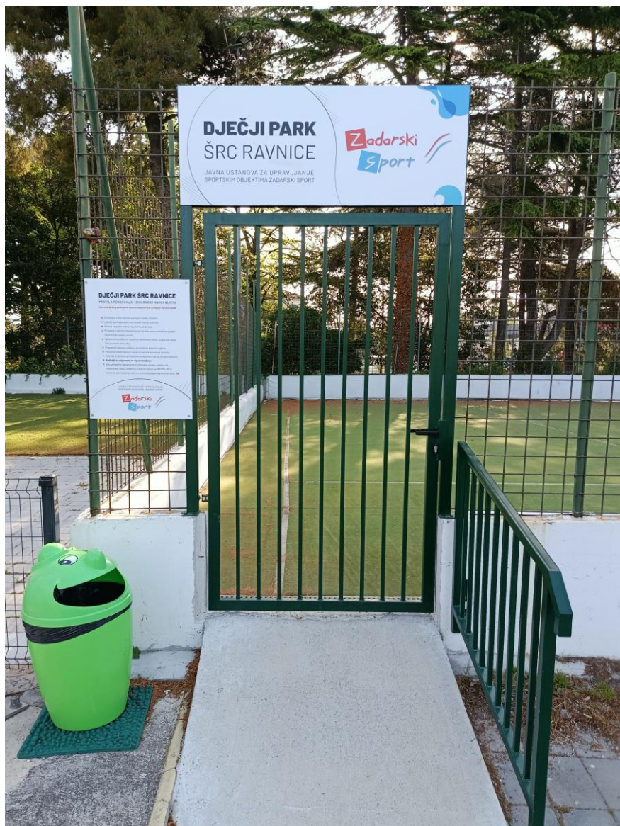
Slika broj 16: Betonska rampa za invalide i dječja kolica te ugrađena metalna ulazna vrata dječjeg igrališta sa bočnim rukohvatom
